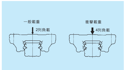
圖 I-5-3 負載狀態
