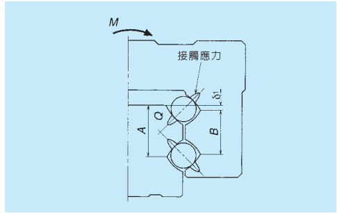
圖 I-5-2 溝槽放大圖（偏移哥德式溝槽）
