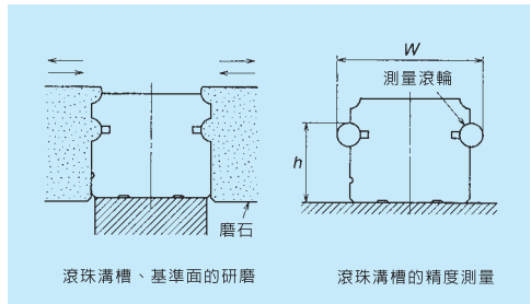
圖 I-5-4 滑軌的研磨和測量
